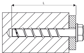
BSZ-SU A4
